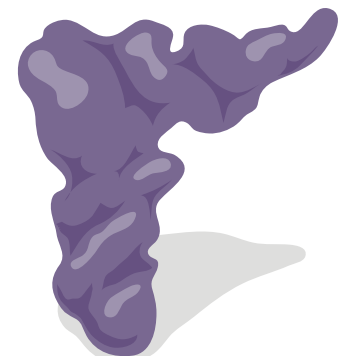
tRNA
